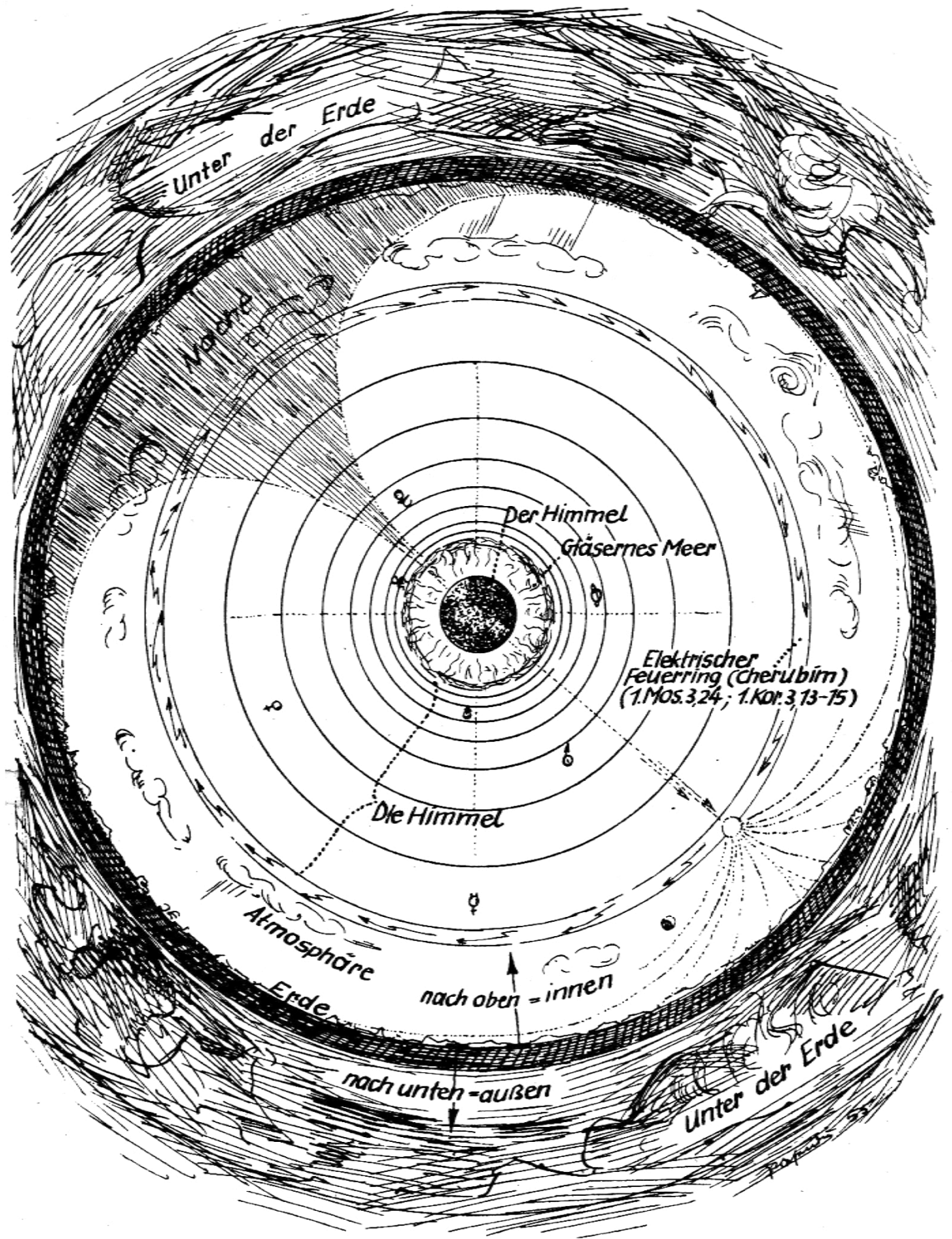
Doorsnede van het heelal
