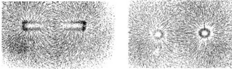
Magnetische veldlijnen. Links: magnetisch spectrum van een staafmagneet. Rechts: magnetisch spectrum van twee ongelijknamige polen.
